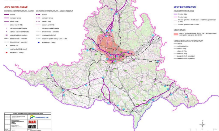
ZÁSADY ÚZEMNÍHO ROZVOJE JIHOMORAVSKÉHO KRAJE Schéma dopravní infrastruktury 1 : 450 000
