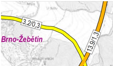
Dopravní model ze studie pro tzv. nulový stav 2035 (v čitateli je celková intenzita, ve jmenovateli intenzita nákladní dopravy v tis. za den)
